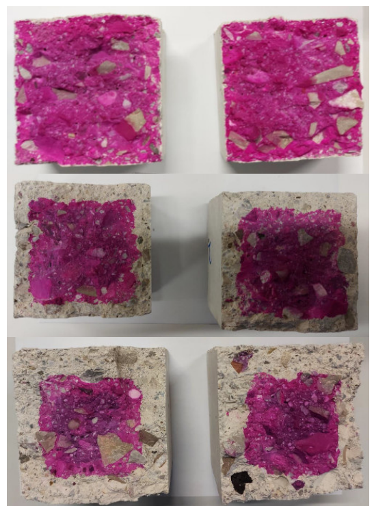
Abb.: Betonlagerung in Kohlenstoffdioxid angereicherter Atmosphäre nach 0, 28 und 70 Tagen
